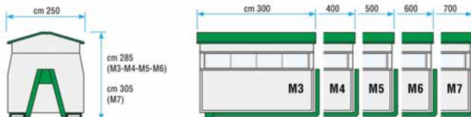
Габариты боен М3—М7
